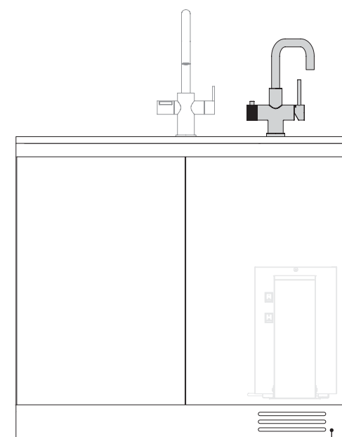
שלושה פתחים בגודל 200x10 מ"מ, או בכל צורה אחרת בתנאי ששטח החורים הינו לפחות 5000 ממ"ר
